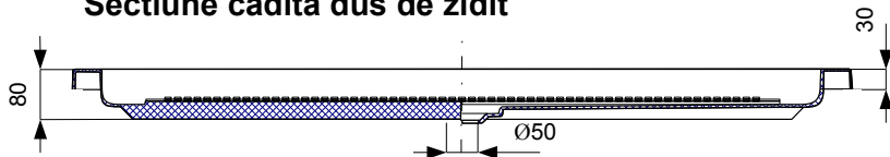
Sectiune cadita dus de zidit
