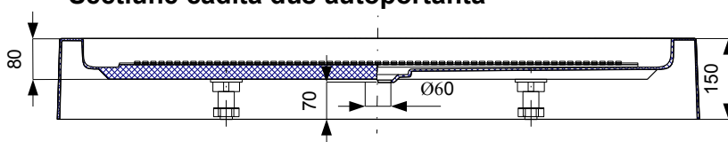
Sectiune cadita dus autoportanta
